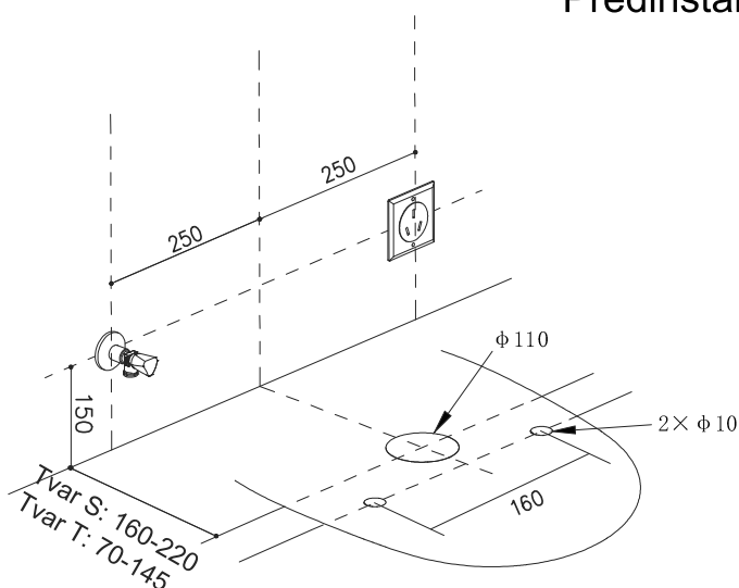
Varianta s odpadem do země
