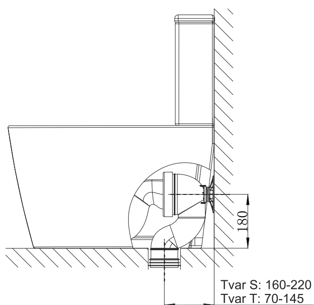
Varianta instalace s odpadem do podlahy
