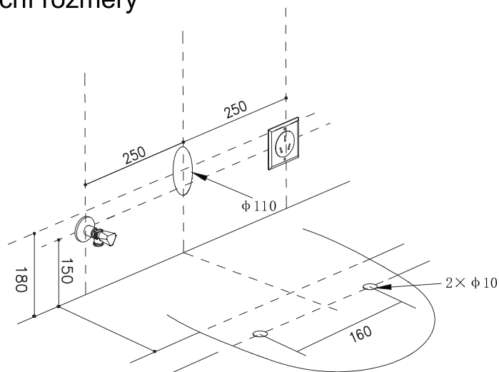
Varianta s odpadem do zdi
