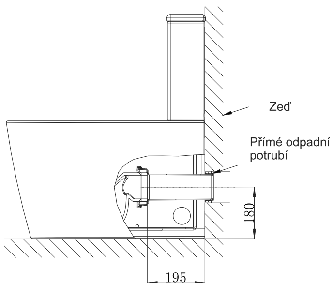
Varianta instalace s odpadem do zdi
