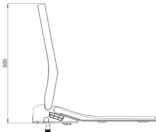
Boční pohled – otevřené víko
