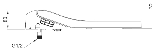
Boční pohled – výška a připojení vody
