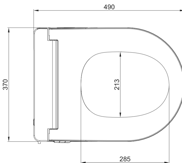
Půdorys – pohled shora
