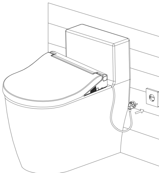
Připojení k elektrické zásuvce
