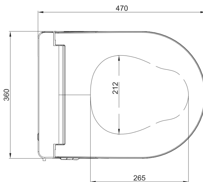
Půdorys – pohled shora
