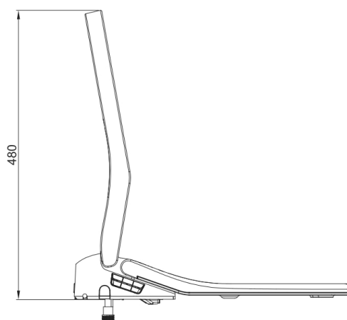
Boční pohled – otevřené víko
