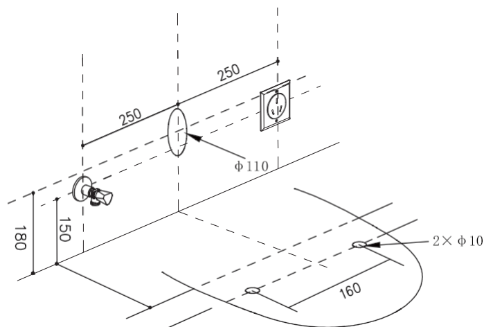
Varianta s odpadem do zdi
