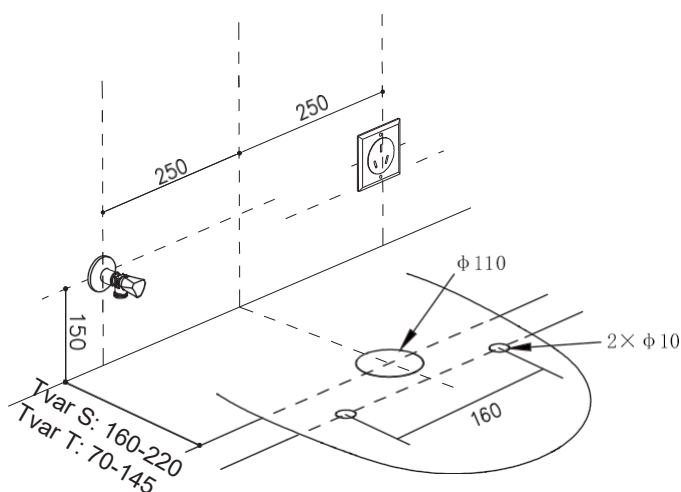
Varianta s odpadem do země
